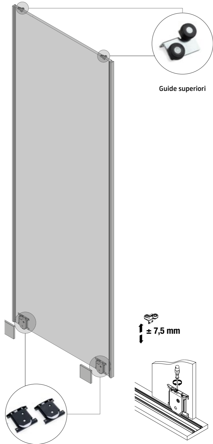
Carrello inferiore
