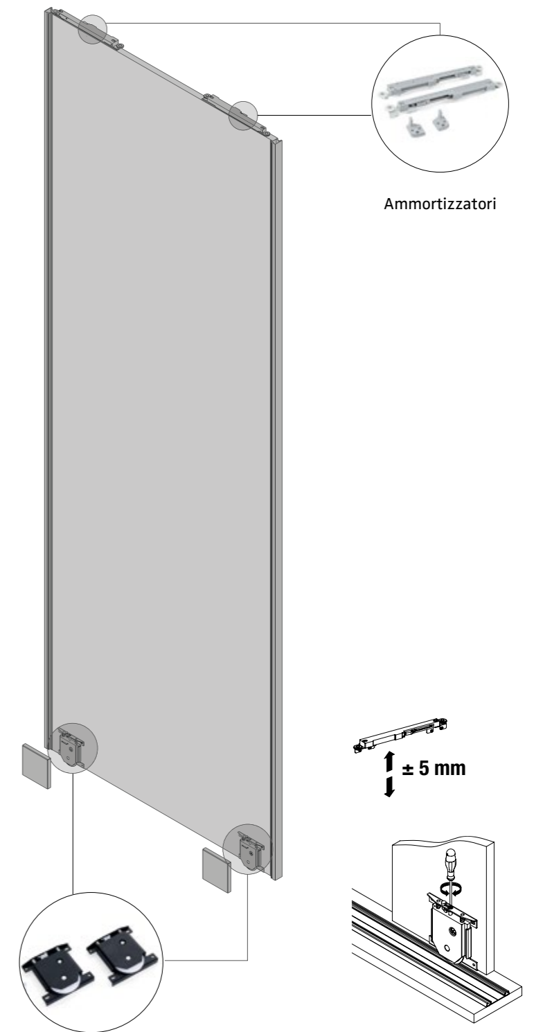
Carrello inferiore
