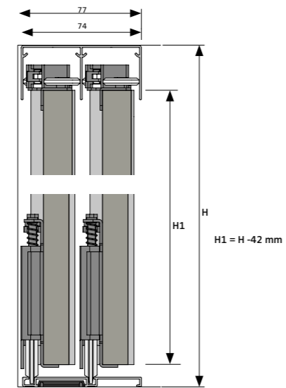
Pannello Legno
